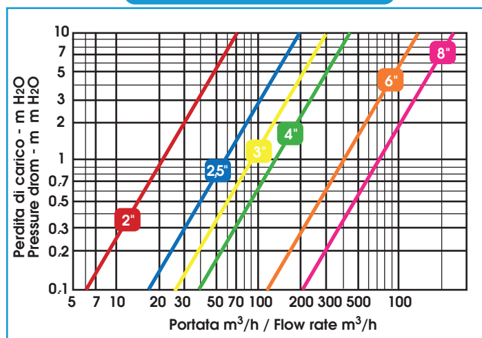
PERDITA DI CARICO / PRESSURE DROP
