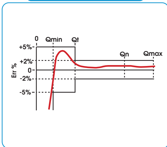
CURVA DI ERRORE / CURVE OF ERROR
